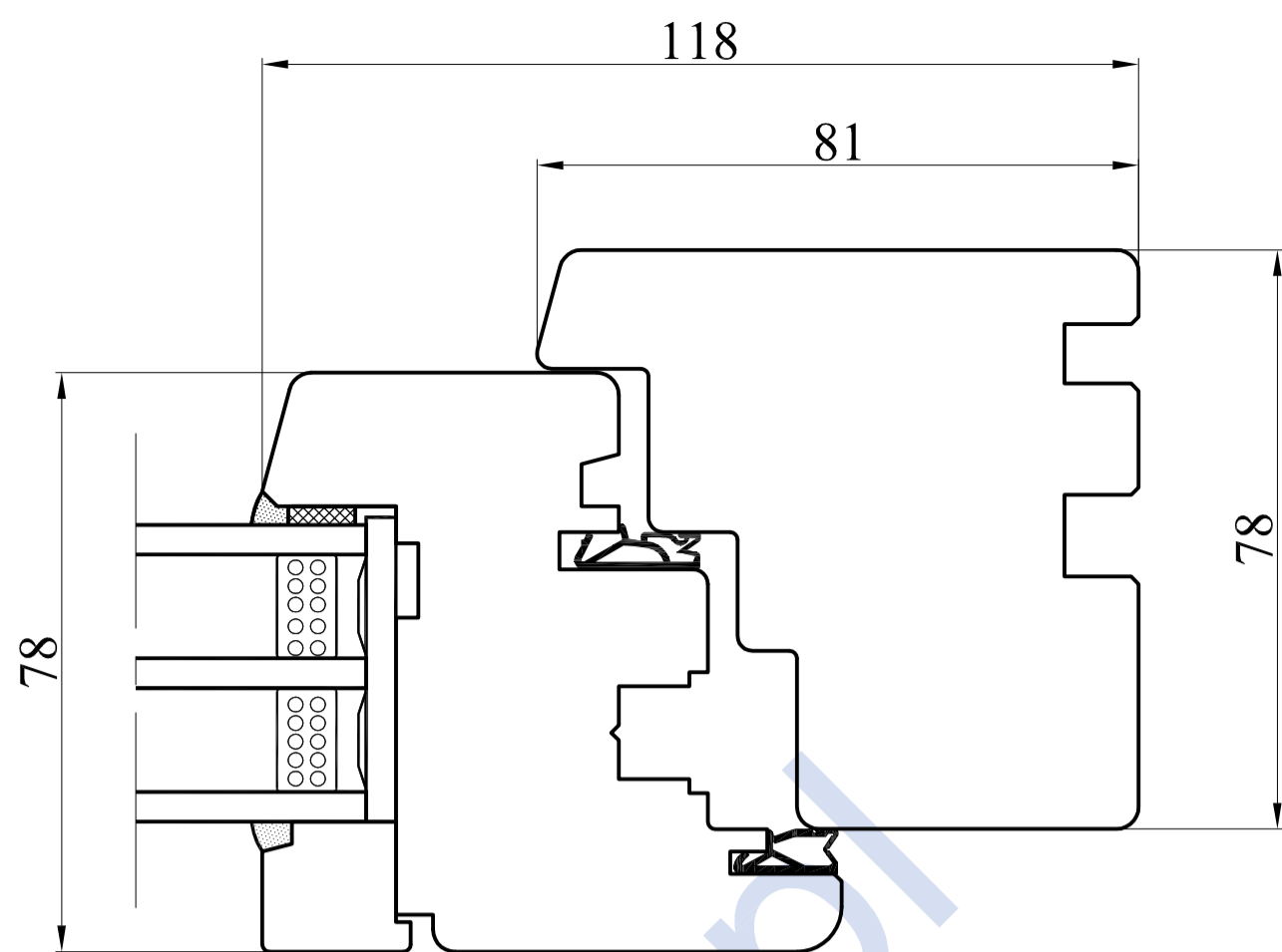
Przekrój B-B
